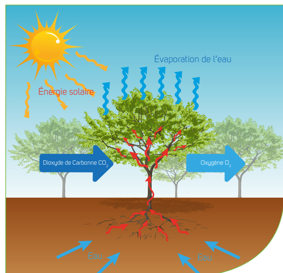
Figure 6 : la photosynthèse
